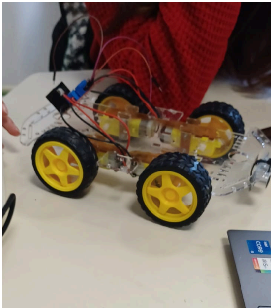
Plataforma con los 4 motores DC del auto a utilizar y Puente H doble L298N.
