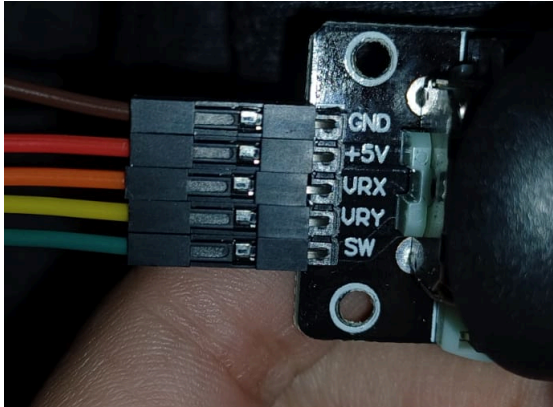
Img 3: Módulo Joystick
