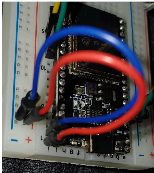
Img 2: Conexiones ESP32
